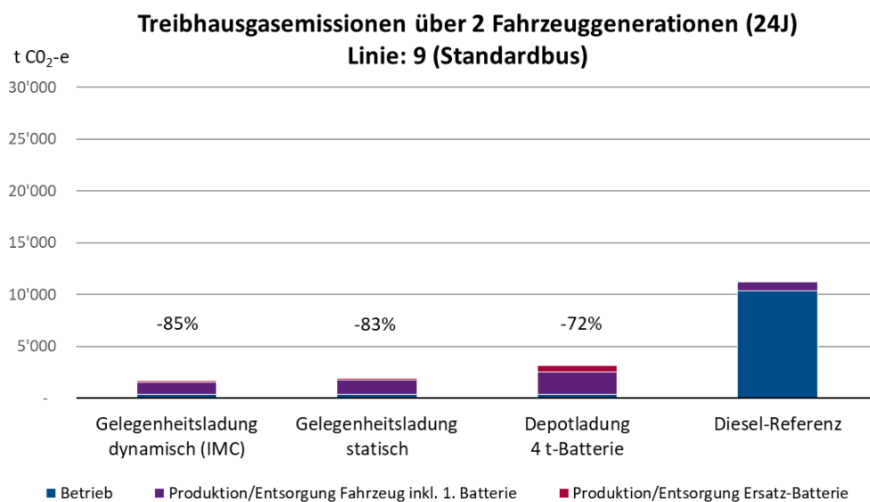
Abbildung 13: Treibhausgasemissionen der drei E-Bus-Varianten und des Dieselsebusses (inkl. Reduktion ggü. dem Dieselsebus in %)
