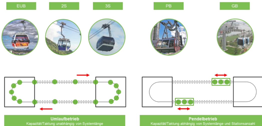
Abbildung 2: Funktionsprinzipien verschiedener Seilbahntechnologien; Quelle: zatran
