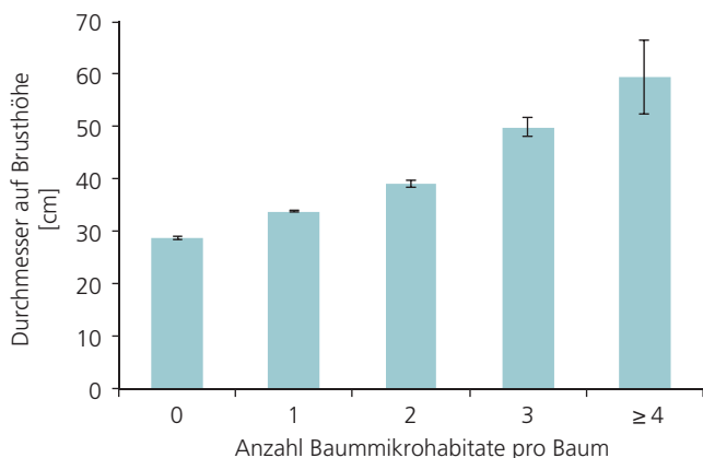
Abb. 3. Nur die dicksten Bäume tragen viele Baummikrohabitate. Mittelwerte mit Standardfehler; alle Unterschiede zwischen den Klassen sind signifikant mit Ausnahme desjenigen zwischen den Klassen «3» und «mindestens 4». Aus BÜTLER und LACHAT 2009.
