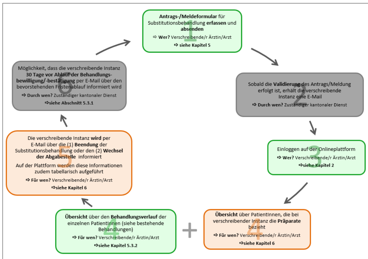
Abbildung 2: Bewilligungs-/Bestätigungszyklus
