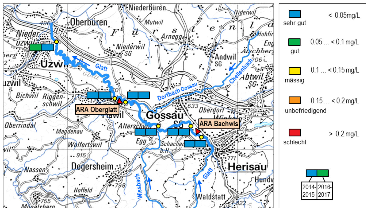
Abbildung 9: \text{NO}_2\text{-N} ; Beurteilung Perioden 2014/2015 (links) und 2016/2017 (rechts); Zustandsklassen gemäss Modulstufenkonzept BAFU (Beurteilungsverfahren: chemisch-physikalische Messgrössen)
