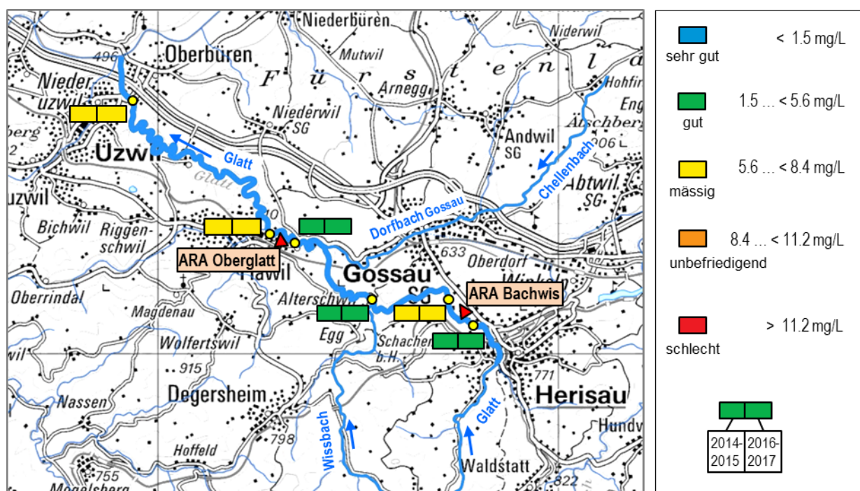
Abbildung 10: \text{NO}_3\text{-N} ; Beurteilung Perioden 2014/2015 (links) und 2016/2017 (rechts); Zustandsklassen gemäss Modulstufenkonzept BAFU (Beurteilungsverfahren: chemisch-physikalische Messgrössen)
