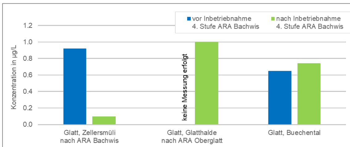
Abbildung 23: Resultatübersicht Benzotriazol, Korrosionsschutzmittel.
