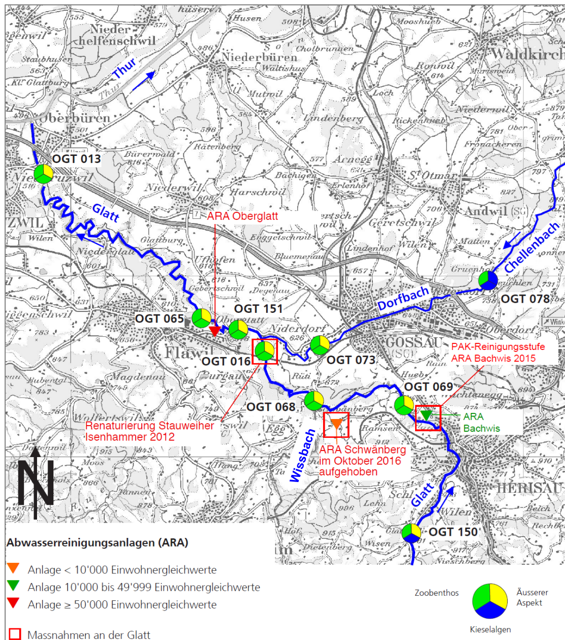
Abbildung 26: Bewertung der untersuchten Stellen an der Glatt, am Dorfbach Gossau und am Chellenbach anlässlich der Untersuchung von 27./28. Feb. 2017 gemäss Modulstufenkonzept BAFU (Module Makrozoobenthos, Kieselalgen, Äusserer Aspekt)
