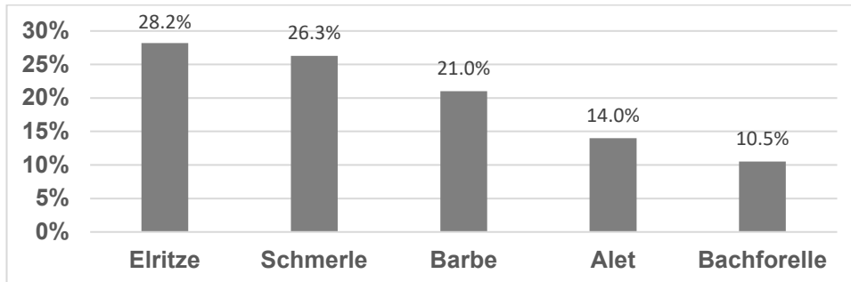
Abbildung 28: Verteilung der gefundenen Arten, Trend-Abfischung 22.09.2015, Glatt Buechental
