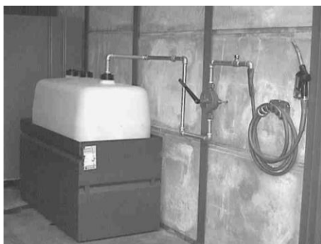
Kleintankanlage
