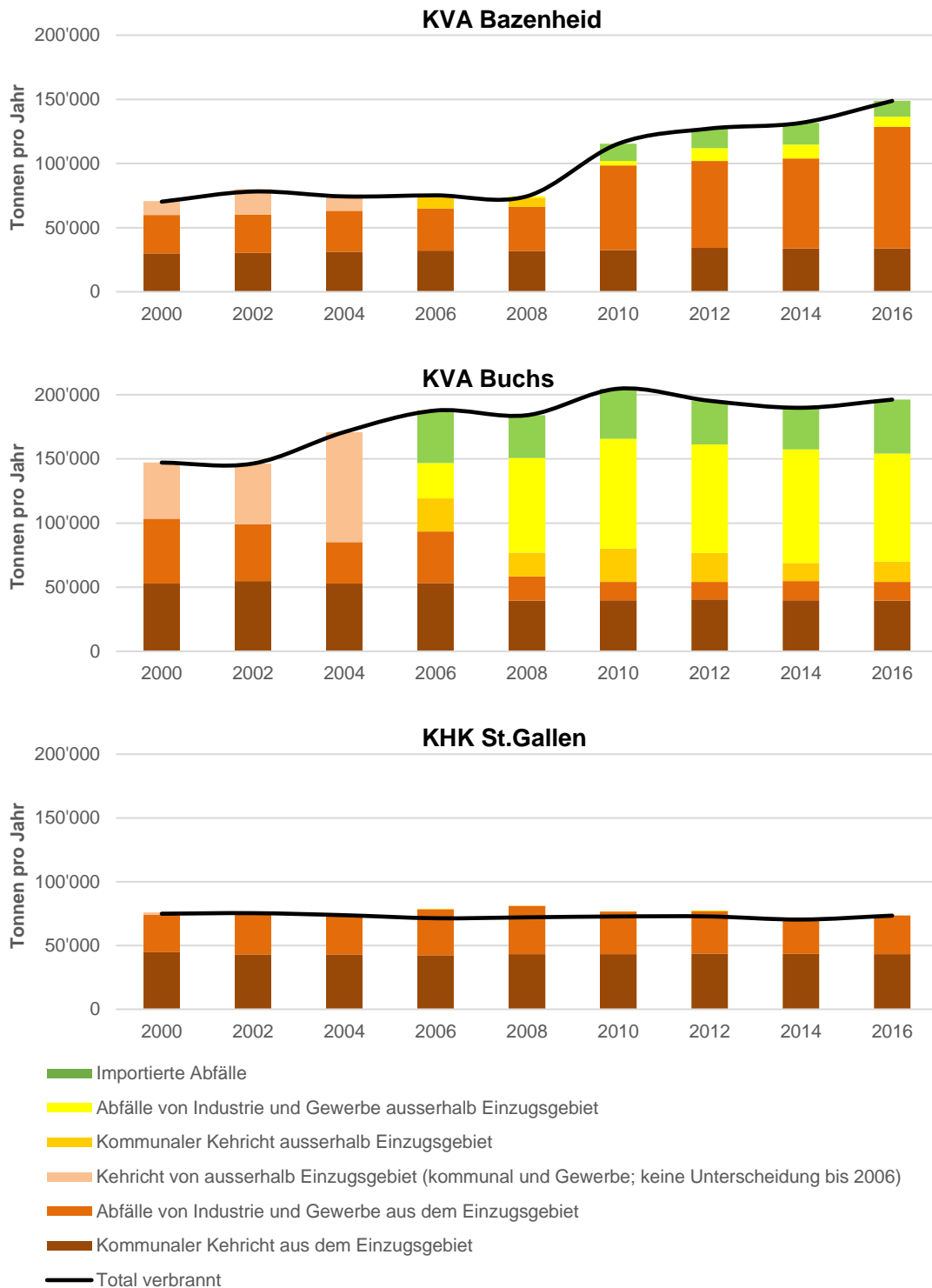
Abbildung 25: Verbrannte Abfallmengen in den Kehrichtverbrennungsanlagen Bazenheid, Buchs und St.Gallen (2000-2016)
