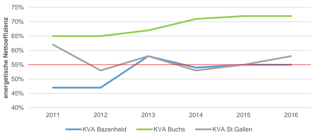
Abbildung 26: Energetische Nettoeffizienz der St.Galler KVA (2011-2016)
