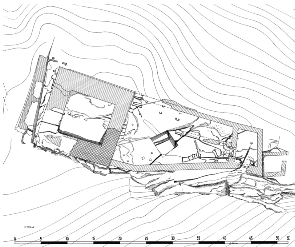
10: Grundrissplan der freigelegten Burganlage, Stand 18. Dezember 1937. Darin eingezeichnet sind neben den Mauerzügen auch der im Zentrum des Burghofs liegende vier-eckige Zisternenschacht sowie die in die Fels Oberfläche gehauenen Fundamentsätze, Balkenlager und Wasserrinnen. Der Verlauf der Höhenkurven mit Äquidistanz 1 m widerspiegelt den Zustand vor den Ausgrabungen.
