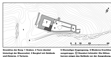
Grundriss der Burg: 1 Graben, 2 Turm (Hochturm), 3 Burghof mit Gebäude, 4 Torturm, 5 Ehemaliger Zugangsweg, 6 Moderne Erschliessungstreppe, 7 Standort Infotafel. Die Höhenkurven zeigen das Gelände vor der Ausgrabung.
