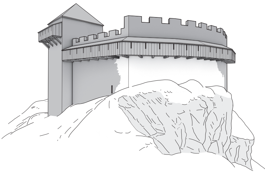
Turm von Südosten. Möglicher Zustand nach einer durch einen Brand der oberen Stockwerke bedingten Reparatur (1316 oder kurz danach), mit reparierter Zugangslaube zum Hocheingang und neu vorgehängter Wehrlaube. Ergänzte Elemente sind dunkel eingefärbt.
