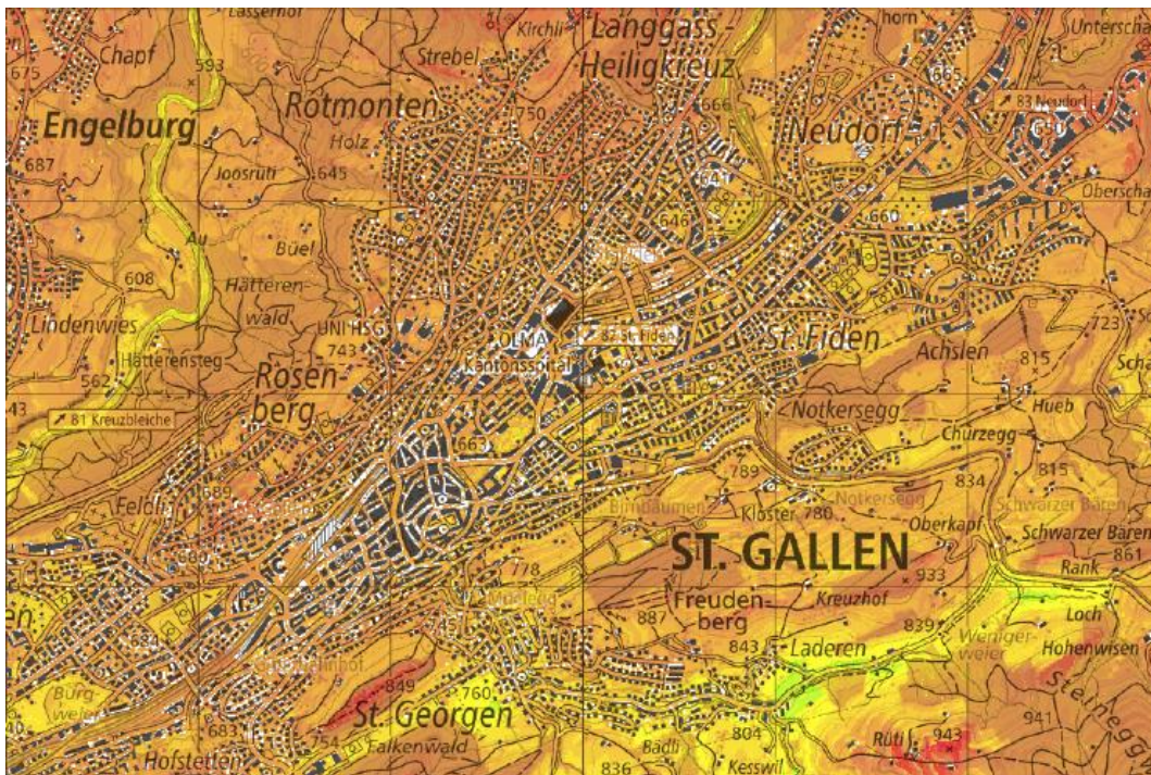
Abbildung 9: Ausschnitt der Klimaanalysekarte der Nachtsituation mit Darstellung der Lufttemperatur.
