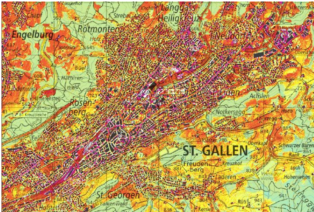
Abbildung 6: Ausschnitt der Klimaanalysekarte der Tagsituation mit Darstellung der PET.
