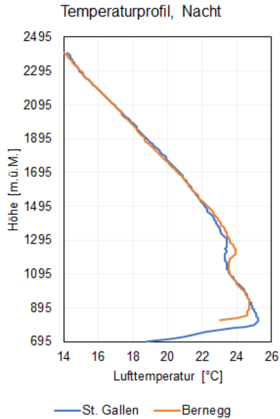
Abbildung 8: Nächtliches Temperaturprofil in St. Gallen und dem Bernegg aus den Modellergebnissen.
