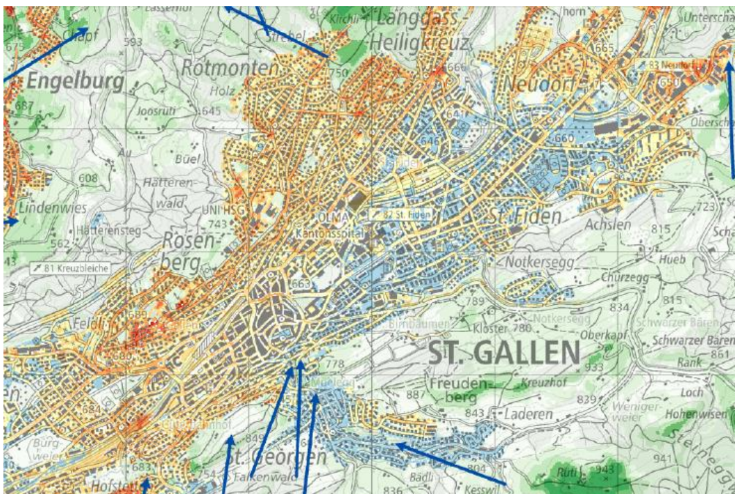
Abbildung 11: Ausschnitt der Klimaanalysekarte der Nachtsituation mit Darstellung der nächtlichen Überwärmung, der Kaltluftvolumenstromdichte und den Kaltluftleitbahnen.
