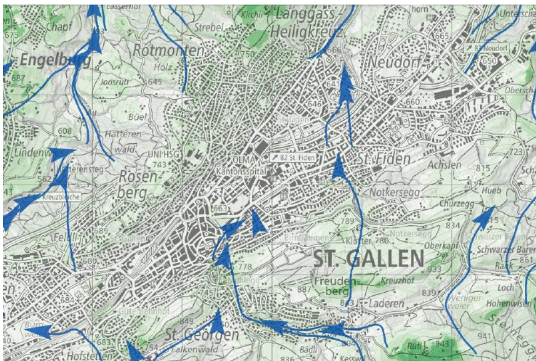
Abbildung 10: Ausschnitt der Klimaanalysekarte der Nachtsituation mit Darstellung des Strömungsfeldes und der Kaltluftvolumenstromdichte.
