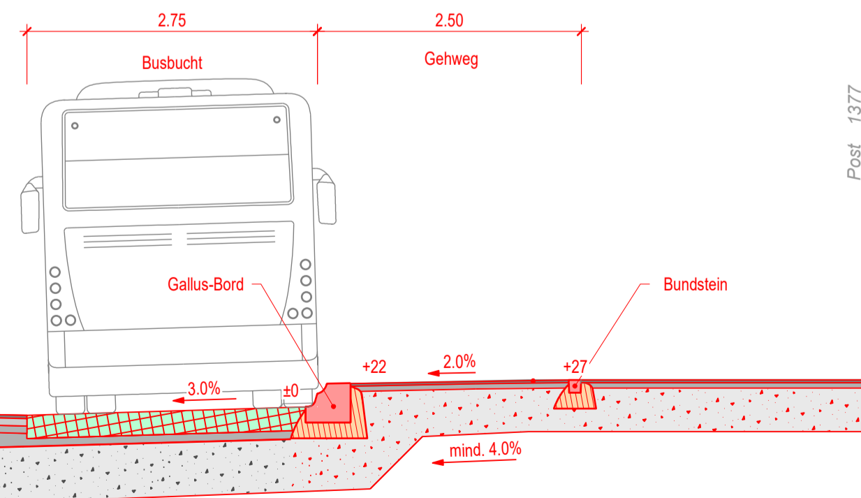
Oberbau Gehweg
