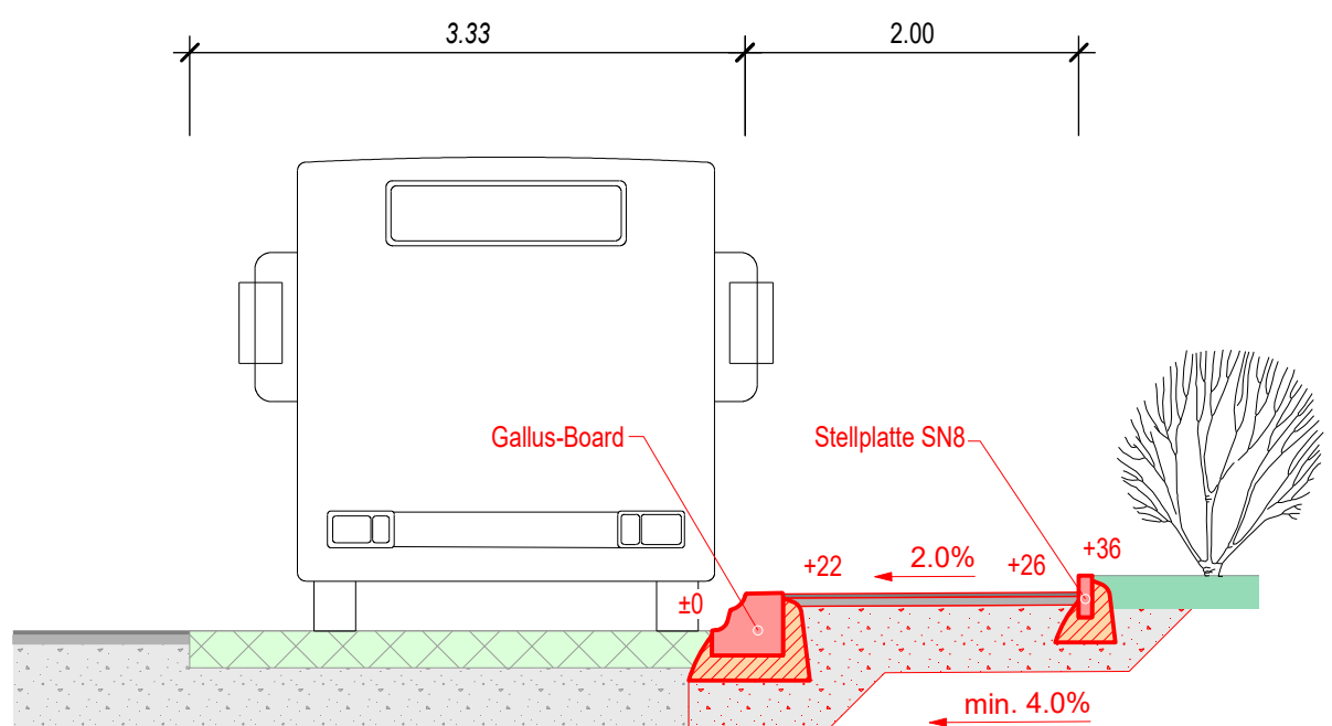
Normalprofil 1:50
