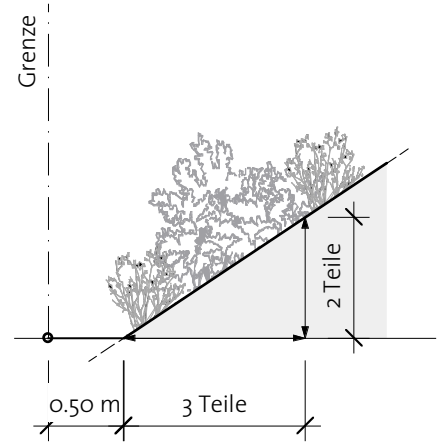
bepflanzte Böschung
