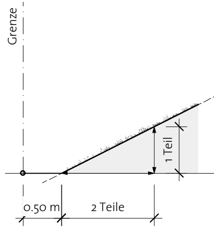
angesäte Böschung
