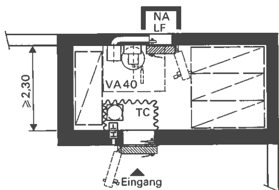
Figur 2.4-5 Grundrissform für 10 Schutzplätze (Bodenfläche \geq 11 m 2 )
